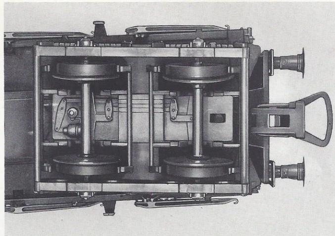
Detail vom Fahrgestell Modell 2025 (Seite 18)
