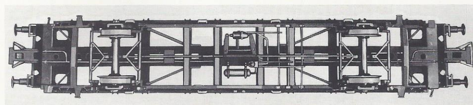
Detail vom Container-Tragwagen 2011 (Seite 17)
