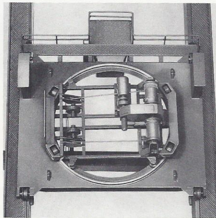
Detail der verschieb- und schwenkbaren Bühnenteile
